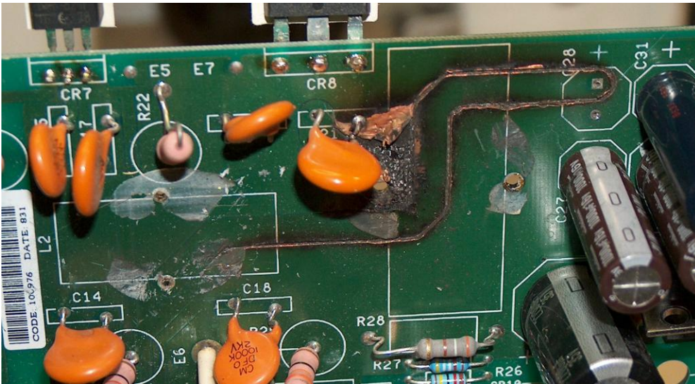
IGT Power supply
